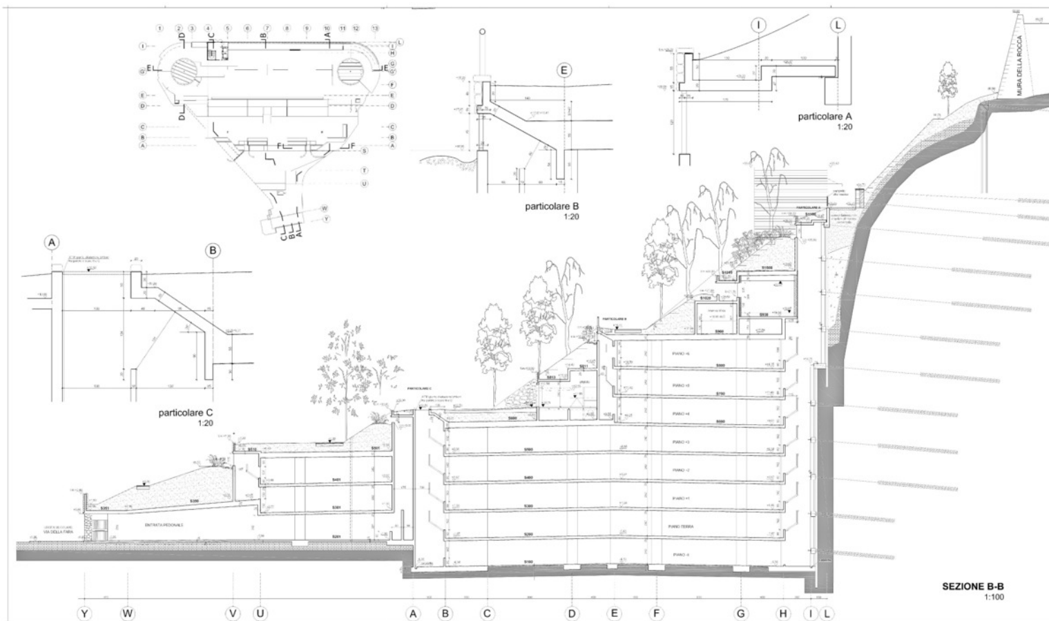
Progetto di Variante in corso d'opera n.1, elaborato 714-EA20 sezione B-B
